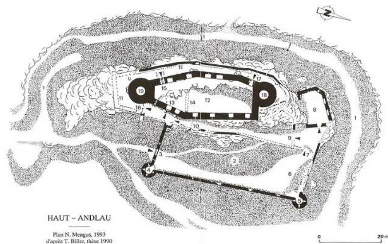
Plan du château du Haut-Andlau
